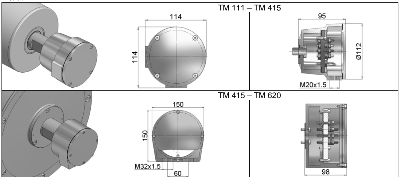
Typ(e) A: Klemmenkasten / terminal box
