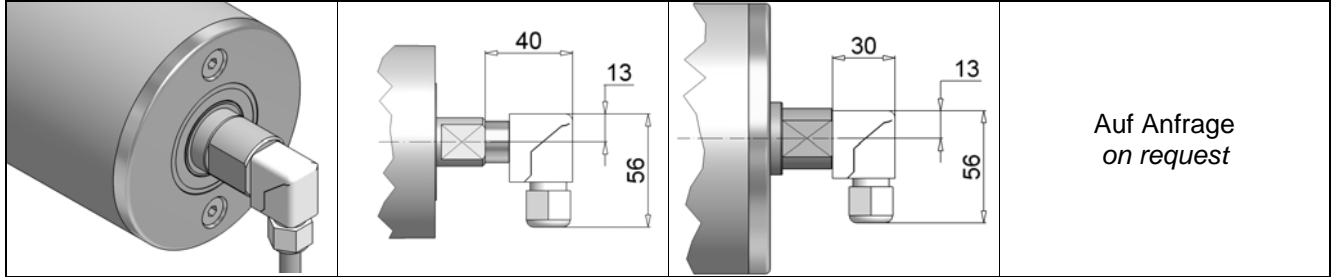
Typ(e) C: Variable Kabelauführung, Zugentlastung innenliegend mit 1m Kabel / variable cable design, pull release inside with 1m cable
