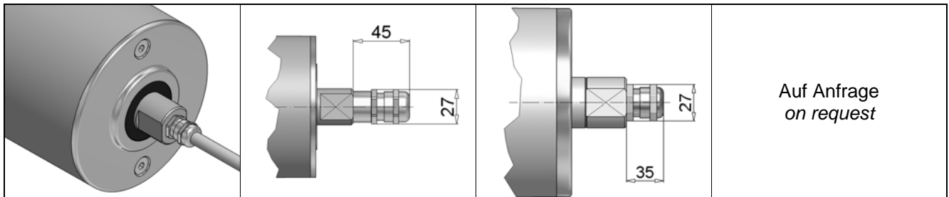
Typ(e) D: Kabelverschraubung gerade mit 1m Kabel / straight cable connection with 1m cable
